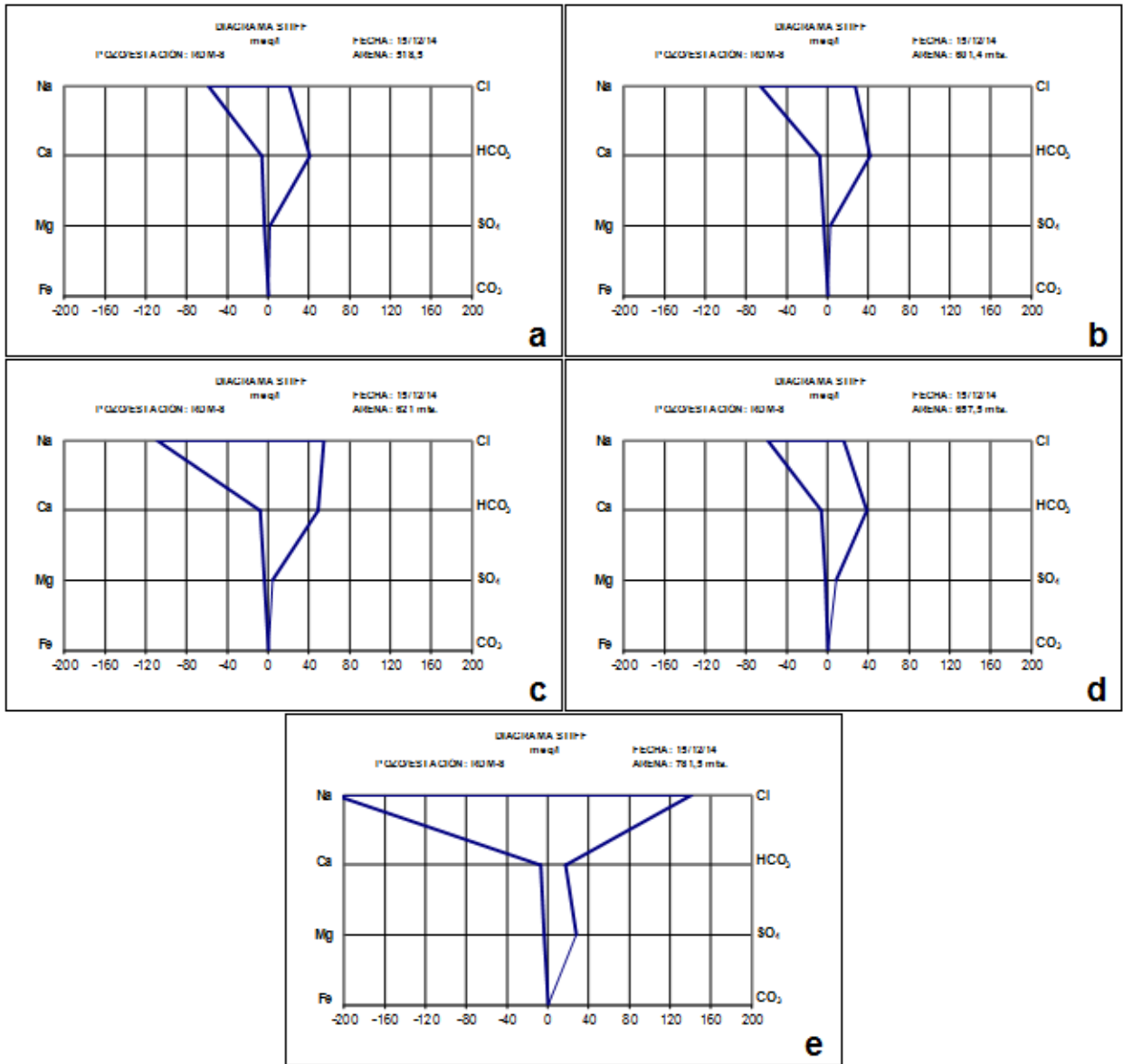
Figura 14: Gráficos de Stiff correspondientes a las muestras obtenidas de capas acuíferas atravesadas por el pozo YPF.Nq.RDM-8 en las profundidades: 518,5m (a); 601,4m (b); 621m (c); 657,5m (d); 781,5m (e).
