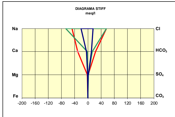
Figura 13: Comparación entre el promedio de las muestras de aguas someras (342m - 508m) con la muestra de agua de 515,5m y el promedio del lodo en el pozo YPF.Nq.RDM-28(d).
