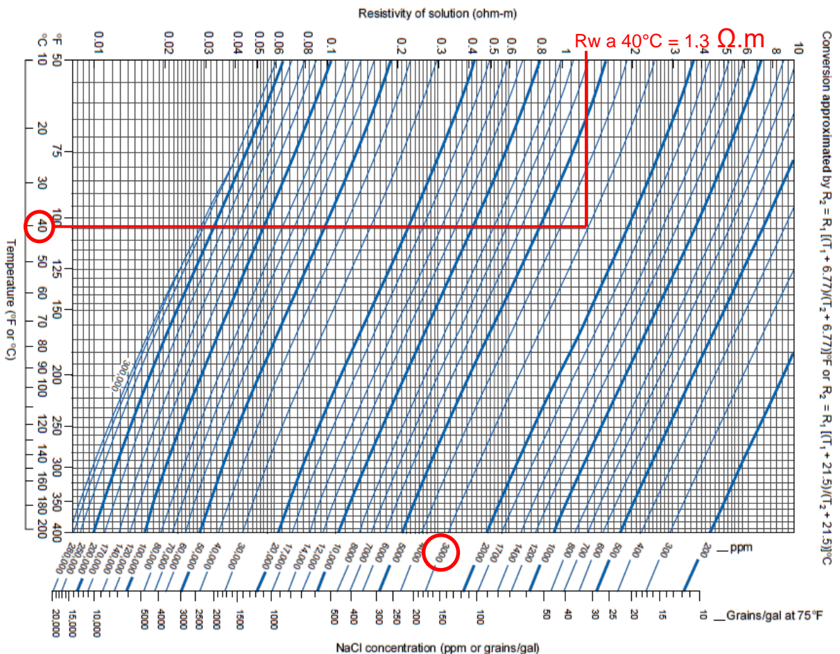
Figura 6: Gráfico Resistividad vs Temperatura en Soluciones de NaCl (Tomado de Schlumberger).
