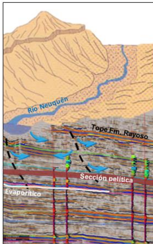
Figura 27: Esquema propuesto de infiltración de agua del río Neuquén a través de fallas semiverticales hacia capas de la Fm. Rayoso.
