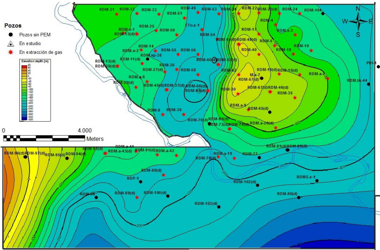
Figura 8: Mapa de profundidades máximas de acuíferos dulces en el área de Rincón del Mangrullo.
