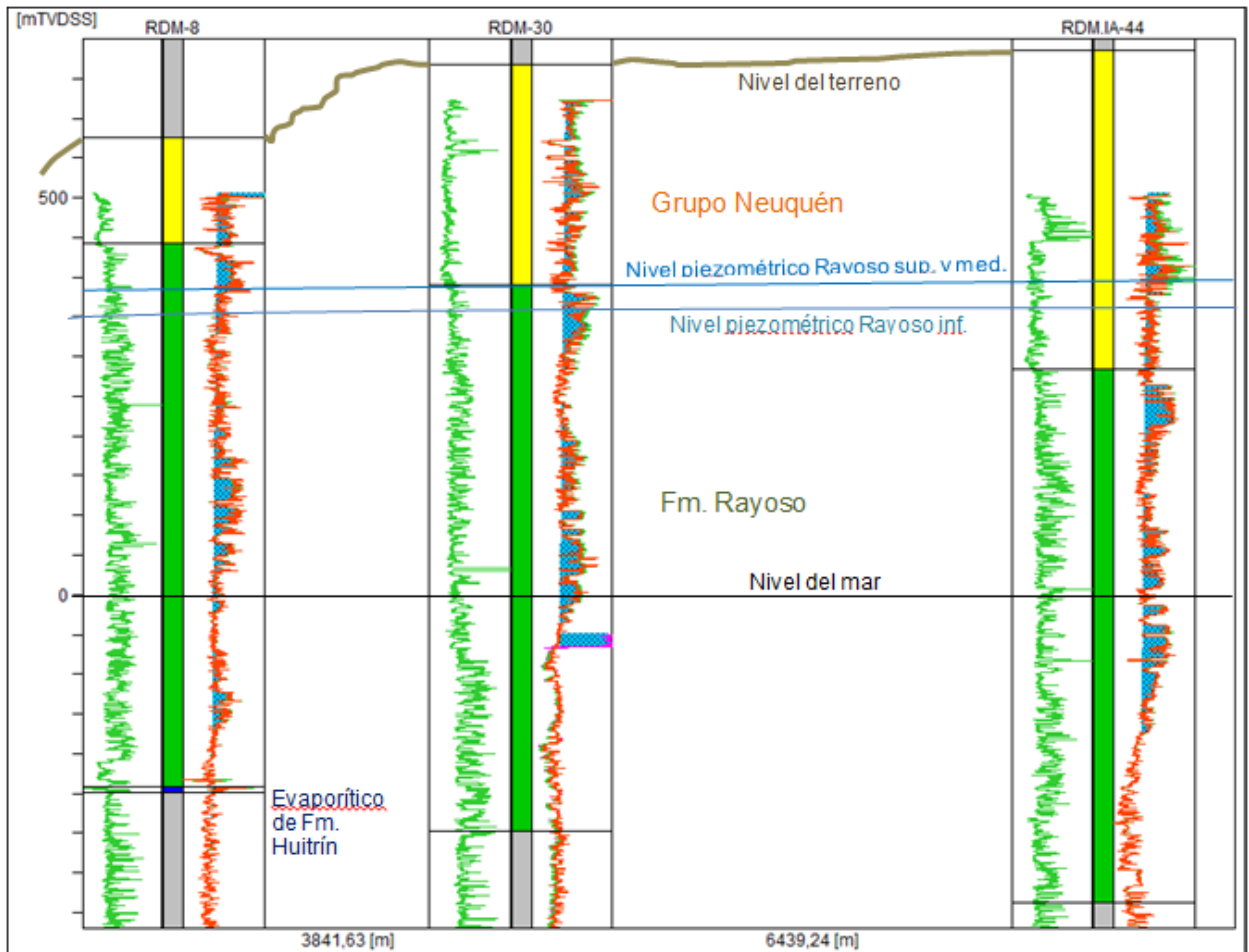
Figura 25: Corte con los niveles piezométricos de la Fm. Rayoso.
