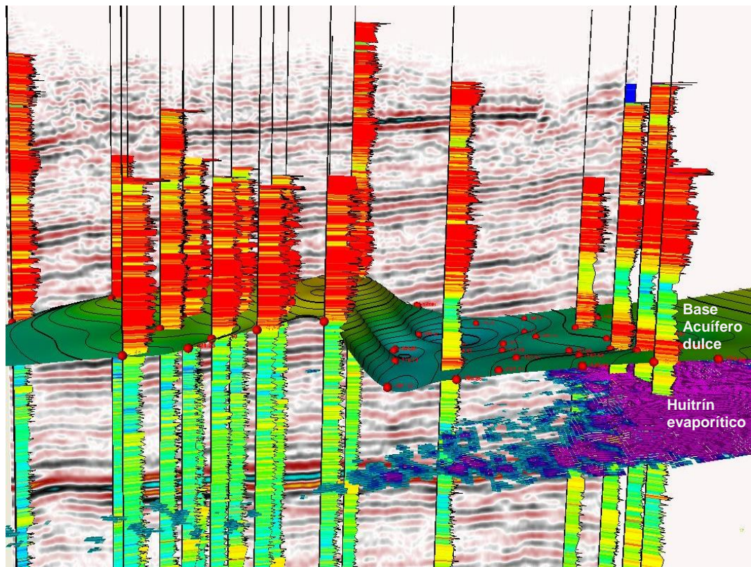
Figura 22: Niveles de base de los acuíferos dulces de Rincón del Mangrullo y su relación con las facies evaporíticas de la Fm. Huitrín.
