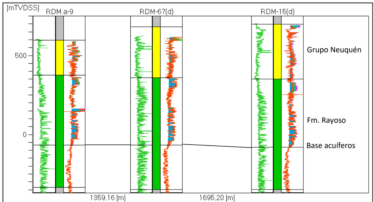
Figura 7: Corte estratigráfico de pozos de RDM con curva cut-off de resistividad marcando la base de los acuíferos dulces.
