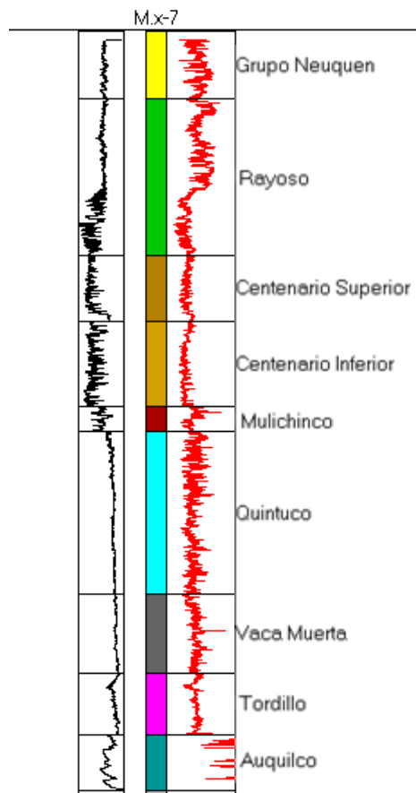
Figura 2: Columna Estratigráfica.
