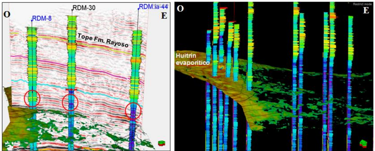
Figuras 20 y 21: Facies evaporíticas y clásticas de la Fm. Huitrín en Rincón del Mangrullo. Puede observarse como la existencia restringida de los acuíferos dulces de la Fm. Rayoso parece estar controlada por la presencia de las facies evaporíticas.
